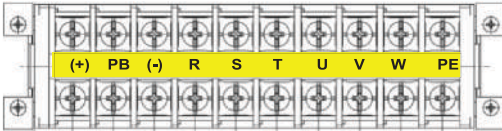
Şekil C-2 4-5.5kW modellerin kablolama terminalleri
