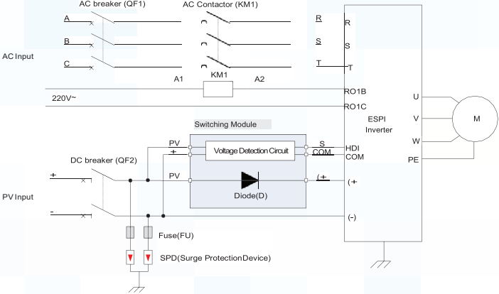
Şekil C-1 İnvertör şebeke & PV değişim çözümü
