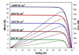
Akım - Voltaj &amp; Güç - Voltaj Grafiği (DI750-132TNB12)
